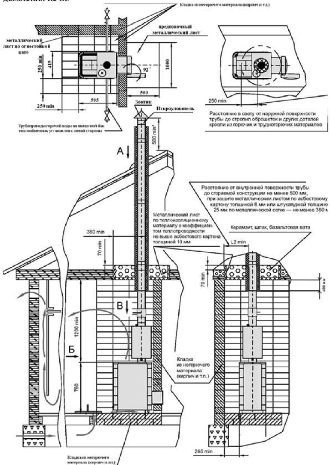
Схема монтажа печи
