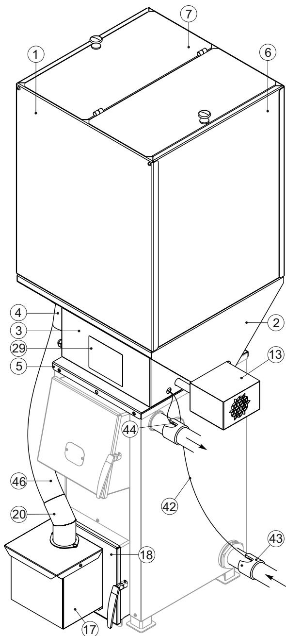
Рис. 1. Конструкция АПГ-25
